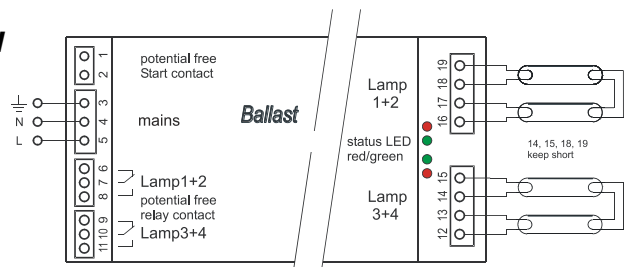
Anschlussbild
